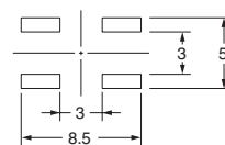
印刷基板焊盘尺寸 (TOP VIEW)
